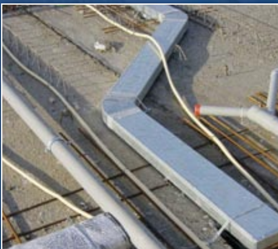
Instortkanalen t.b.v. WTW installatie
