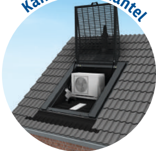
Inschuifbaar frame
